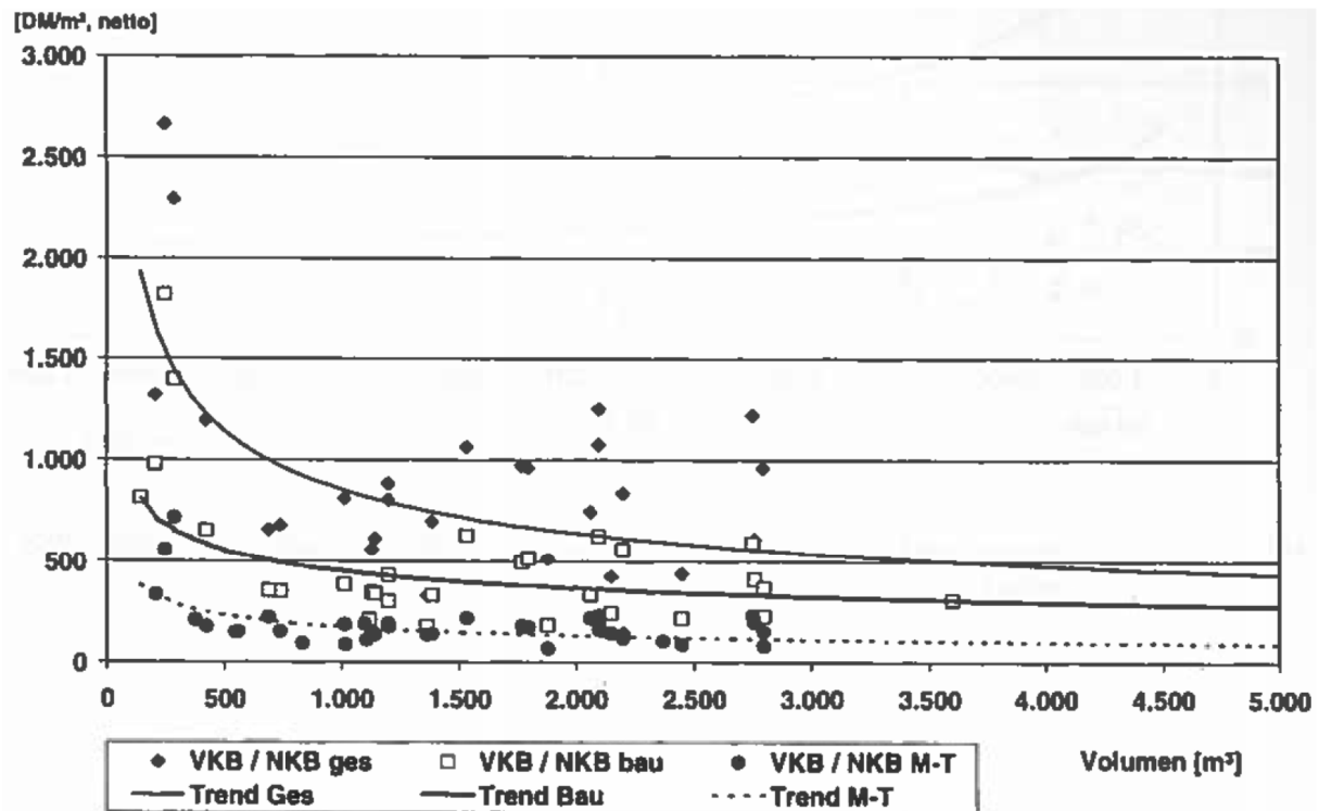
Abbildung 14: Investitionskosten für Sedimentationsbecken (Vor- und Nachklärbecken) (korrigierter Preisindex). [DM/m³, 1999 netto].
